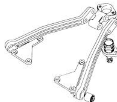
PUENTE TRIANGULAR
